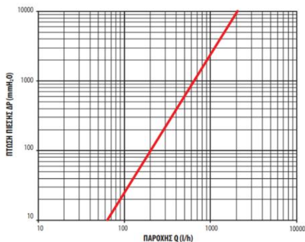
Smart Form • Διάγραμμα Πτώσης Πίεσης
