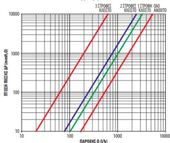
Smart II &amp; III • Διάγραμμα Πτώσης Πίεσης
