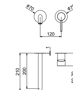
PARTE ESTERNA DA UTILIZZARE SOLO CON CORPO INCASSO 35AC5004 EXTERNAL PART TO BE USED ONLY WITH BUILT-IN BODY 35AC5004
