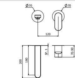
PARTE ESTERNA DA UTILIZZARE SOLO CON CORPO INCASSO 35AC5004 EXTERNAL PART TO BE USED ONLY WITH BUILT-IN BODY 35AC5004
