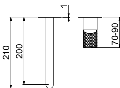
PARTE ESTERNA DA UTILIZZARE SOLO CON CORPO INCASSO 35AC5004 EXTERNAL PART TO BE USED ONLY WITH BUILT-IN BODY 35AC5004
