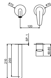
PARTE ESTERNA DA UTILIZZARE SOLO CON CORPO INCASSO 35AC5004 EXTERNAL PART TO BE USED ONLY WITH BUILT-IN BODY 35AC5004
